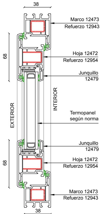
Detalle 1
